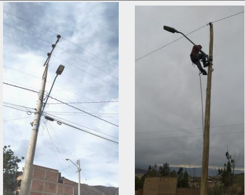
Inst. de luminarias y accesorios de alumbrado público
